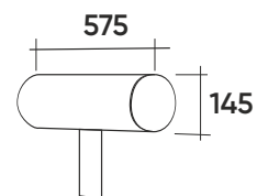
Подголовник Т80
