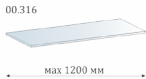
полка стеклянная
