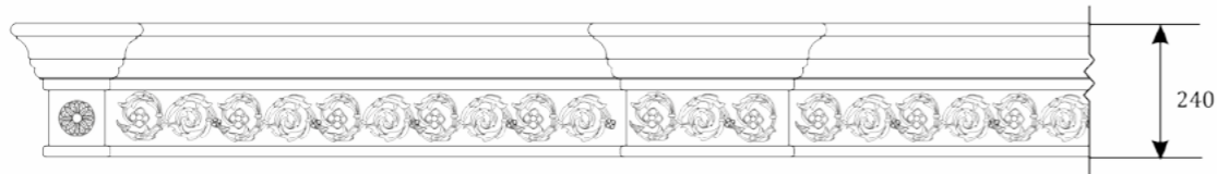
Вариант карниза №2
