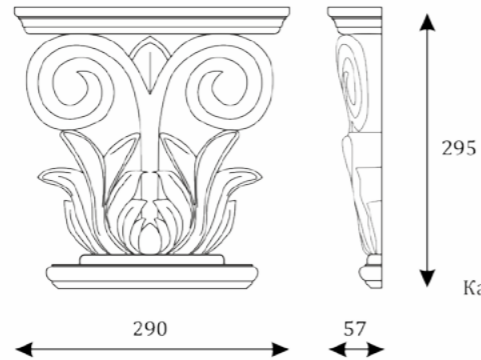
Кронштейн резной.
