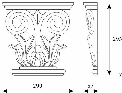
Кронштейн резной.
