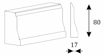
Плитус.
